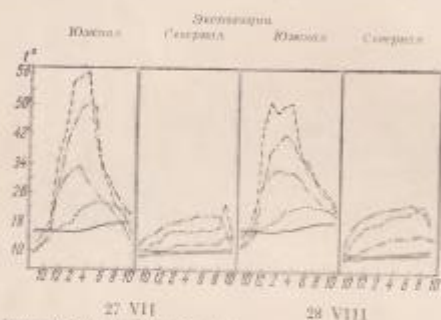
Кривые температуры воздуха: — на высоте 50 см; — на поверхности; — на глубине 3,5 см; — на глубине 10 см; — на глубине 25 см.
